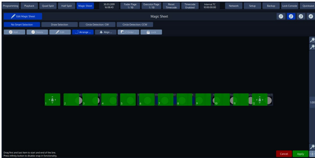
Fig. 183: Arrange Linear
