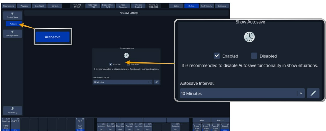
Fig. 40: Show Autosave
