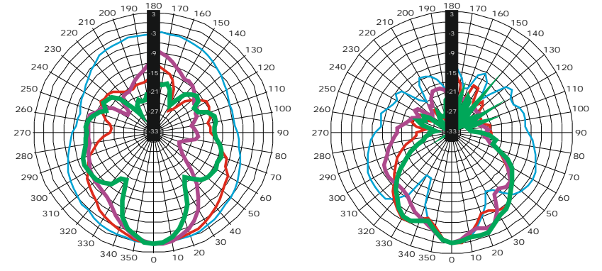
VERTICAL POLAR DIAGRAM — 4000 — 5000 — 6300 — 8000 — 9000 — 10000 — 12500 — 14000
