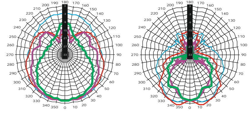
VERTICAL POLAR DIAGRAM — 250 — 500 — 800 — 1000 — 1400 — 2000 — 2500 — 3150
