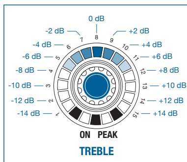
Illustration 21 : Incrémentation de la couronne de DEL de la fonction TREBEL
