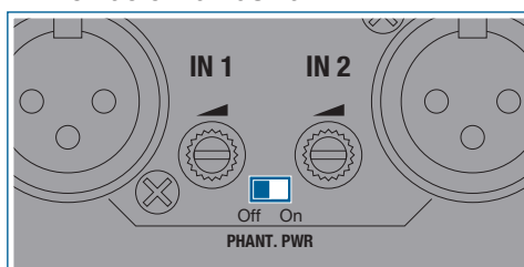
Figura 11: Alimentación fantasma
