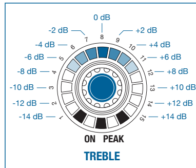
Abbildung 21: Skalierung des LED-Kranzes der Funktion TREBLE
