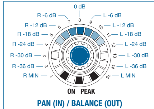
Abbildung 40: Skalierung des LED-Kranzes der PAN / BALANCE Funktion
