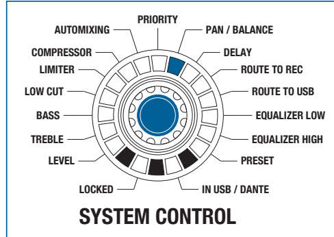
Illustration 39 : Fonction PAN / BALANCE
