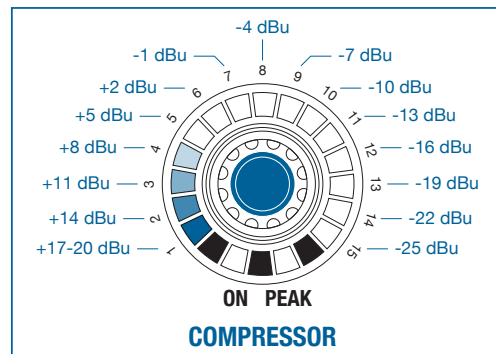
Abbildung 33: Skalierung des LED-Kranzes der COMPRESSOR Funktion
