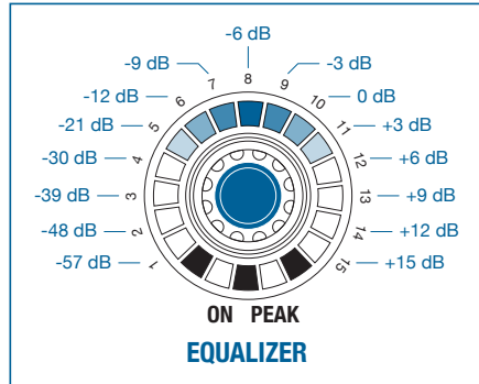
Abbildung 48: Skalierung des LED-Kranzes der EQUALIZER Funktion
