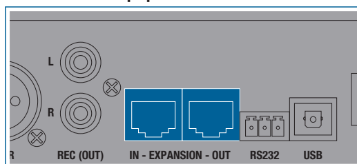
Figura 10: Expansión
