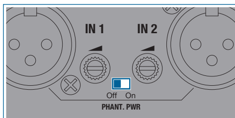
Illustration 11 : Alimentation fantôme
