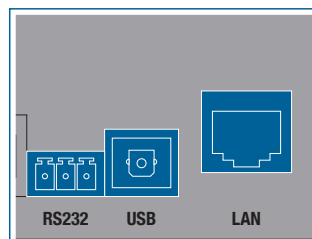
Abbildung 8: USB-Anschluss
