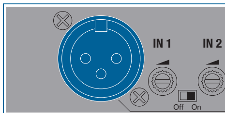
Illustration 3 : Canal d'entrée
