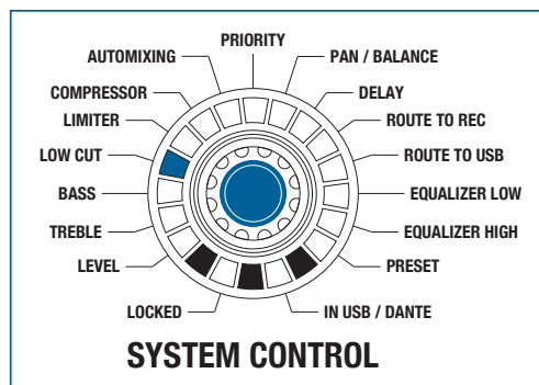
Illustration 26 : Fonction LOW CUT
