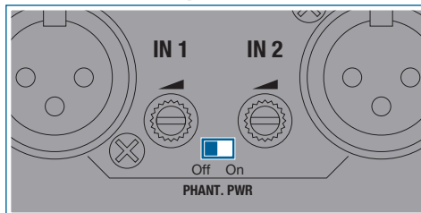
Abbildung 11: Phantomspeisung
