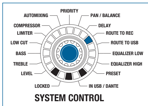
Illustration 43 : Fonction ROUTING TO REC
