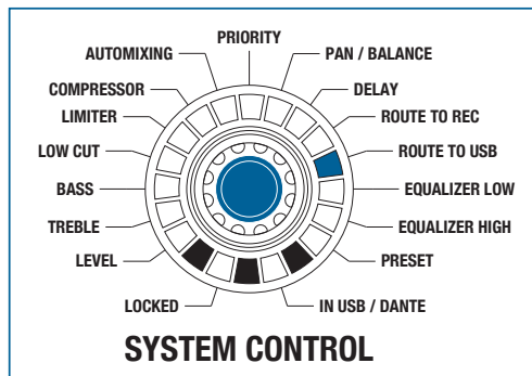
Figura 45: Función ROUTING TO USB
