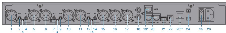
Illustration 2 : Face arrière du DMM8 U (UL, ULD)
