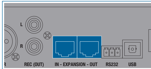
Abbildung 10: Expansion
