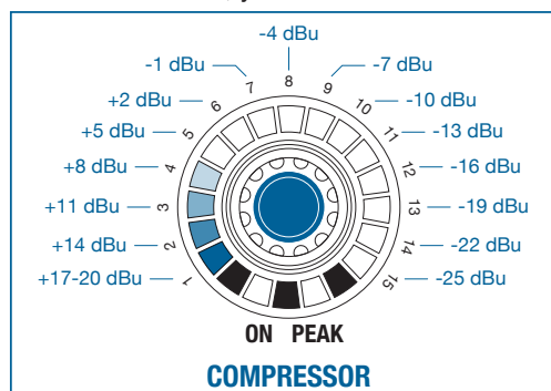
Figura 33: Escala del círculo de LEDs de la función COMPRESSOR
