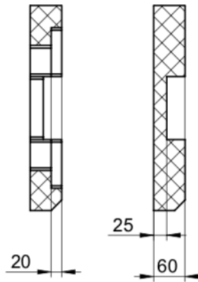
FOAM L-L
